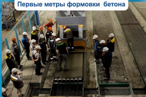
Первые метры формовки бетона
